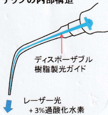
中空型スケーラー チップの内部構造
